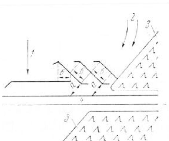
Рис. 10. Расположение снегозащитных заборов на участке дороги у густого леса: 1 — основное направление ветра; 2 — отклоненное от леса направление ветра; 3 — густой лес; 4 — дорога; а — около 15-кратной высоты забора; б — перекрытие (около 10 м)
